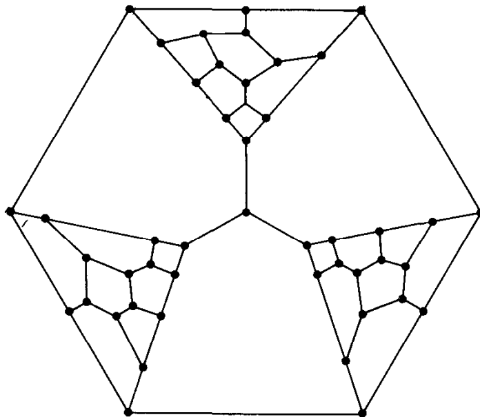
Fig. 7.4. The Tutte graph.
