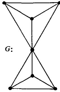
Fig. 10.1. The graph K_4 \cdot K_4 .
