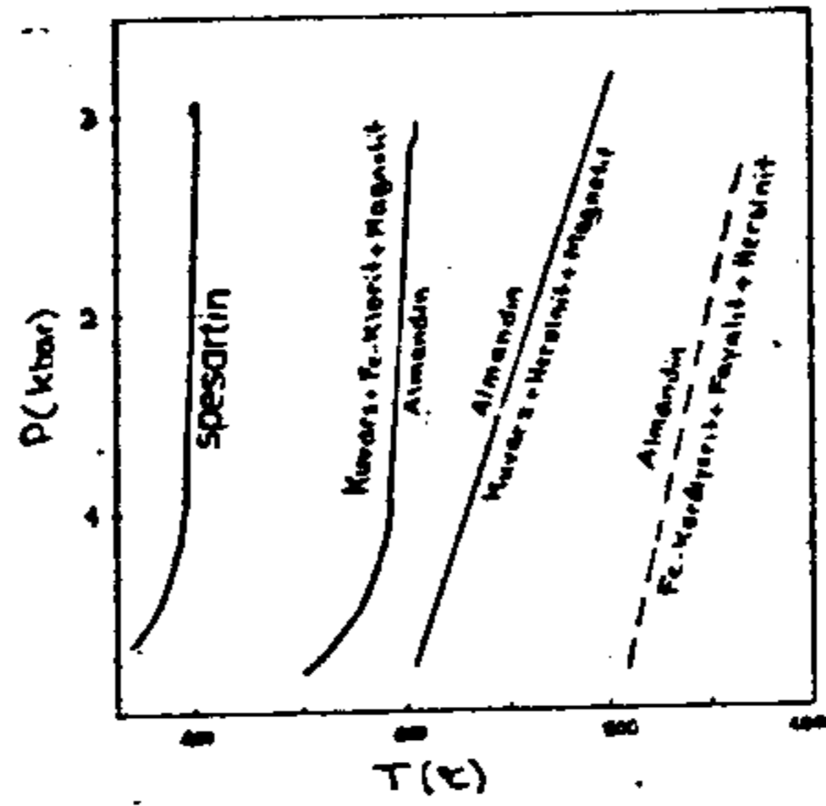
Şekil 8. Çeşitli granatların duraylılık eğrileri (Hsu, 1968).
