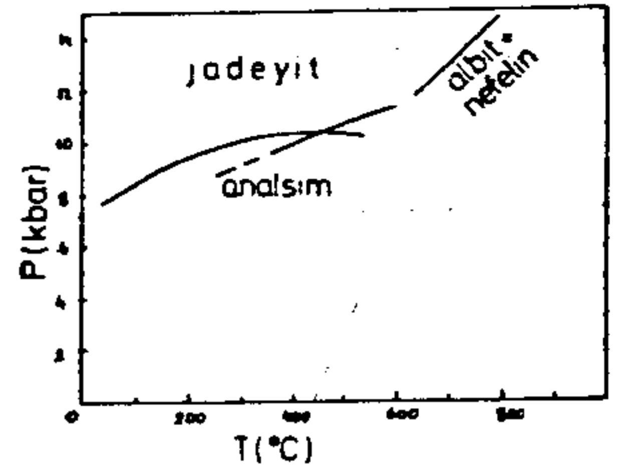
Şekil 7. Jadeyit'in duraylılık koşulları ve dönüşüm eğriği (Newton ve Fyfe 1976).
