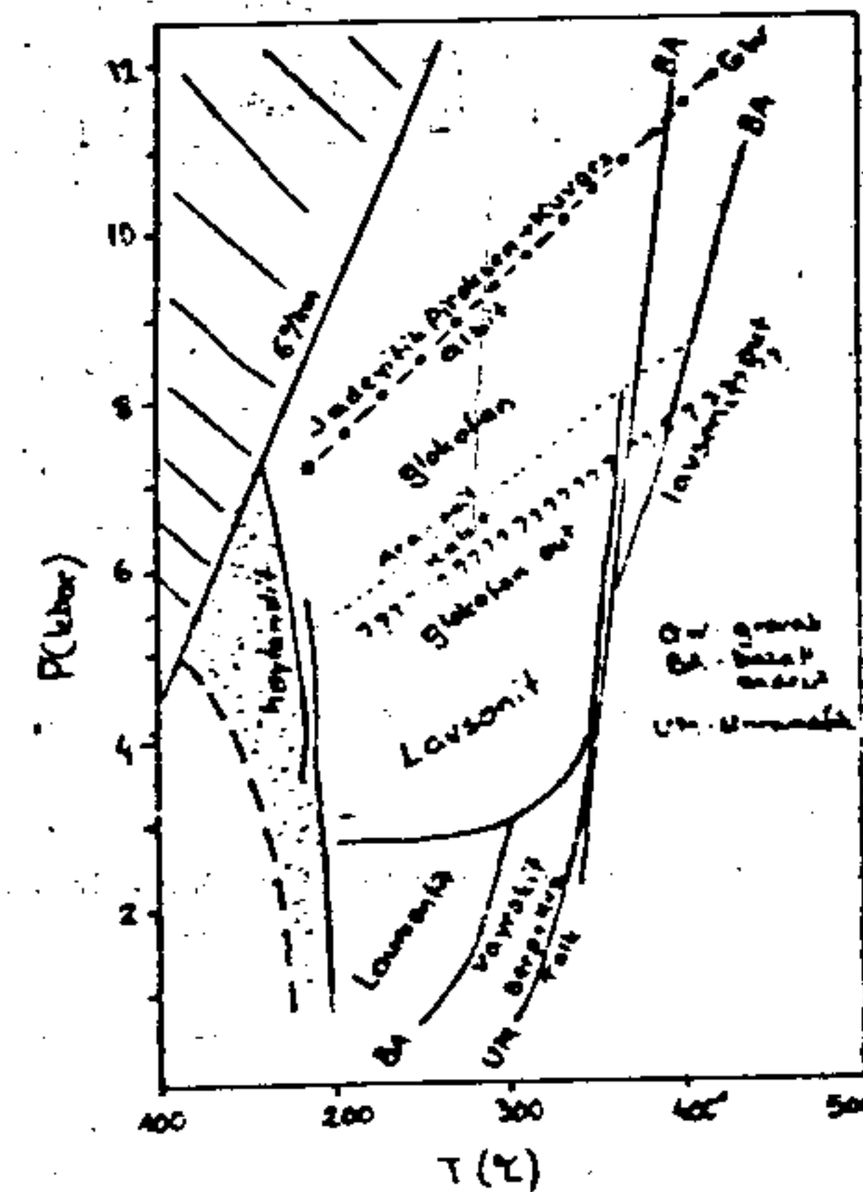
Şekil 10. Winkler (1976)'e göre çok düşük derecedeki metamorfizmanın PT koşulları ve mineral duraylılık eğrileri.
