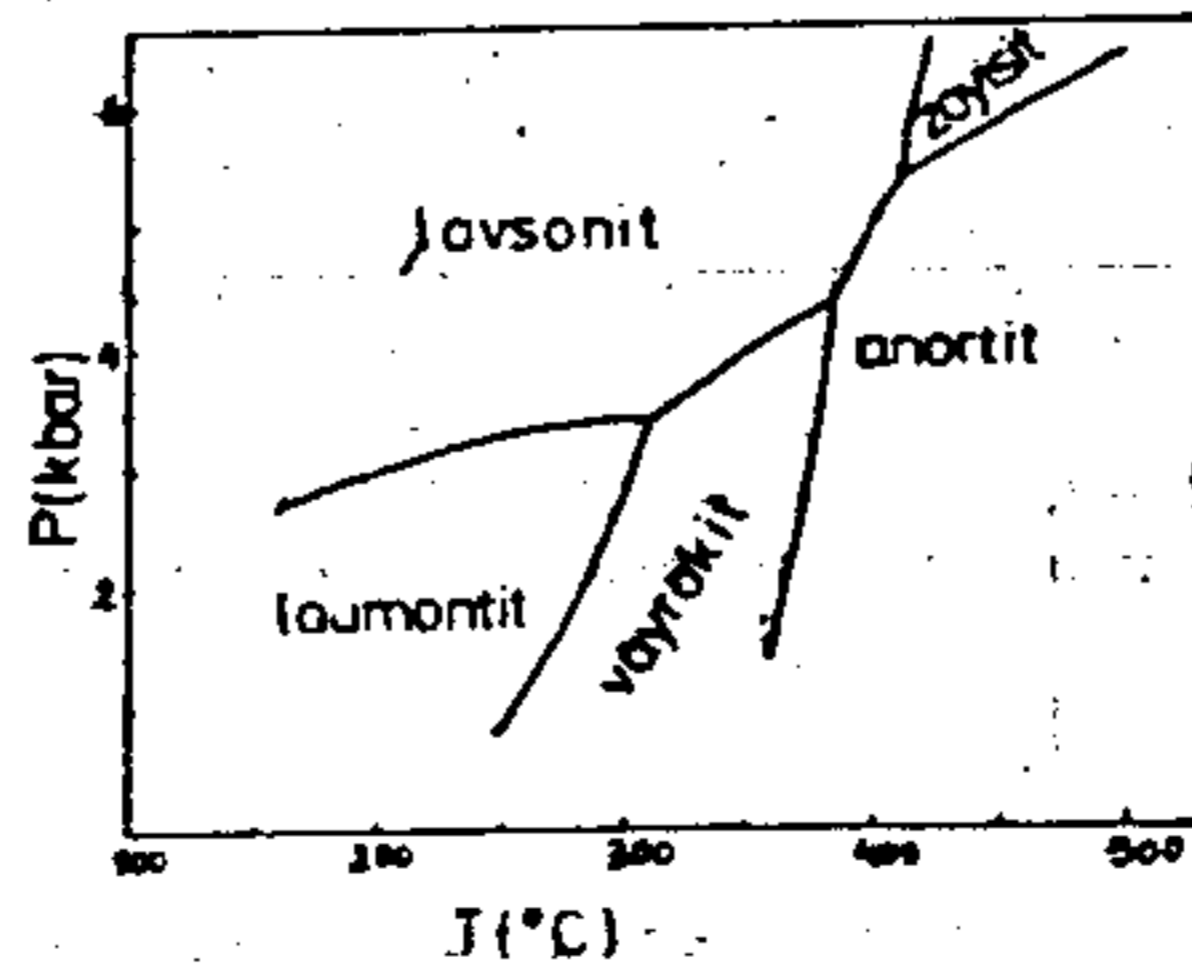
Şekil 6. Lavsonit'in duraylılık alanı ve dönüşüm eğriği (Newton ve Fyfe, 1976)
