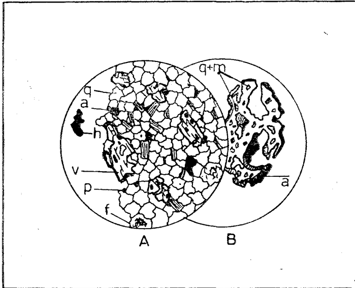
gefil 3: A — Viridin gnaysın mikroskopik görünümü (25x) (a — alümit, b — feldspat, c — hematit, p — piyemontit, q — kuvars, v — viridin). B — Viridin poikiloblastı dış kenarında hematite dönüşmekte ve alargitten oluşma bir tepkime zonu kapsamaktadır, (a — alümit, q — Di — kuvars ve muscovit)
