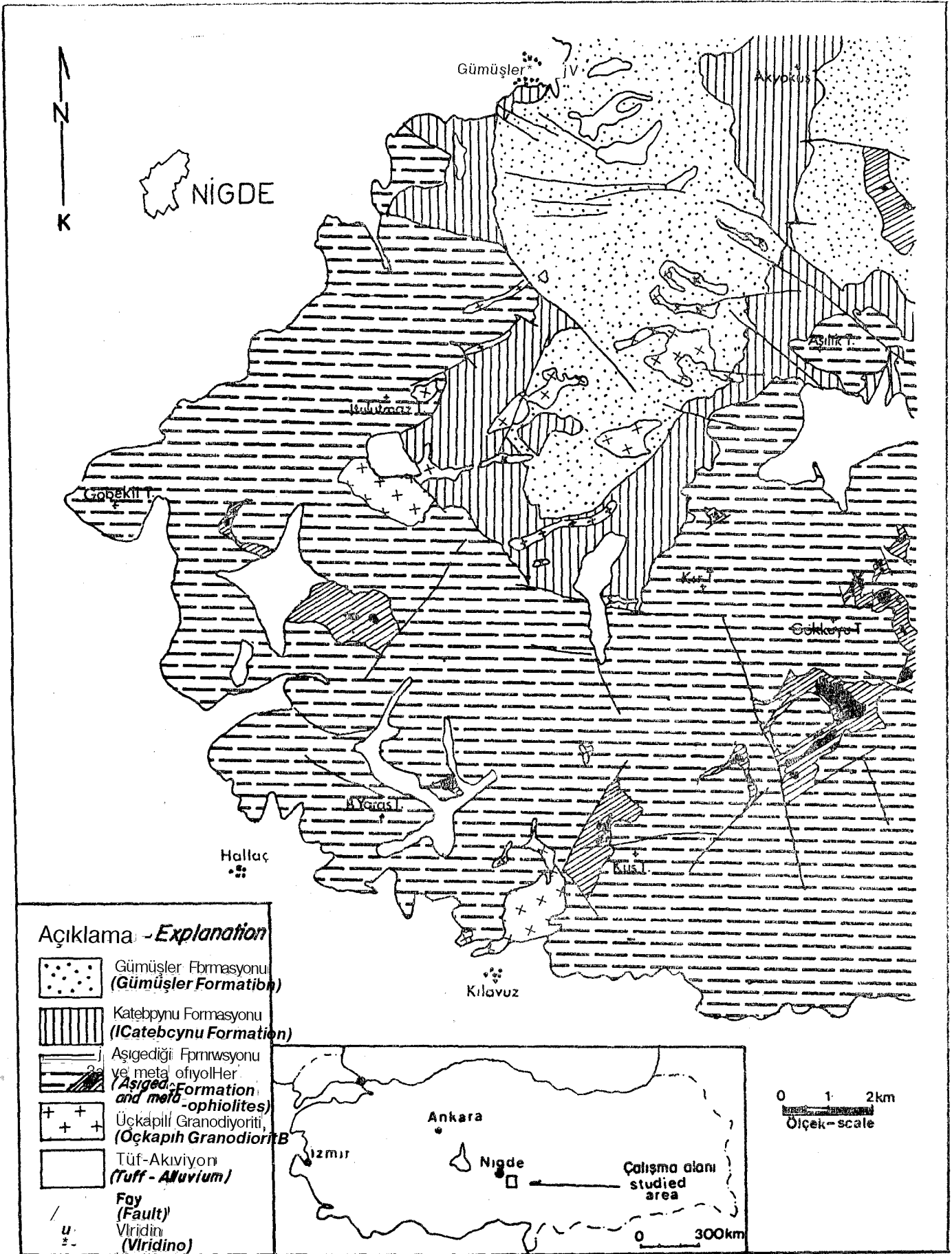
Sekil 1: Niğde Masifi batısının jeoloji haritası (Göncüoğlu, 1977'den sadeleştirilmiştir),
