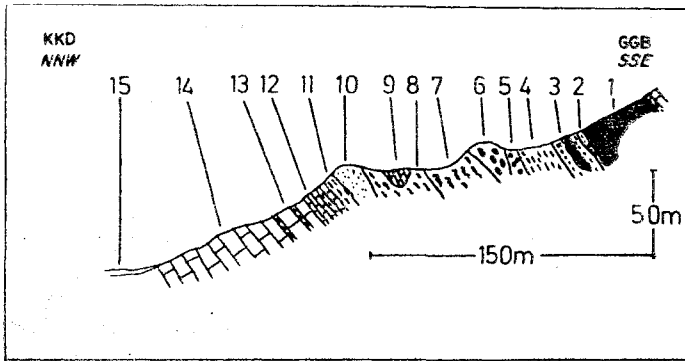
gefil 2: Gökkuyn Tepe kuzey-kuzeydoğusunda viridli gnays içeren metamorfik karmadığın konuma (1. Serpentin, 2. Klorit-serpentin, 3. Grammatit-sist, 4. Kordiyerit-muskovit-jutys, 5. Viridin-gnays, 6. Amfibolit, 7. Amfibol-klorit-fjist, 8. Klorit-gist, 9. İnce taneli mermer, 10. Kuvarsit, 11. Amfibol-kuvarsit, 12. Kalksist, 13. KalksikatU mermer, 14. Mermer, 15. Yamaç moloza).
