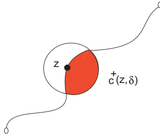
Fig. 3. The region c^+(z, \delta) .
